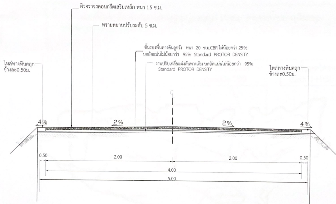
รูปตัดถนนคอนกรีตเสริมเหล็ก ทห 15 ซม. มทจร ๖๓ NO SCALE
